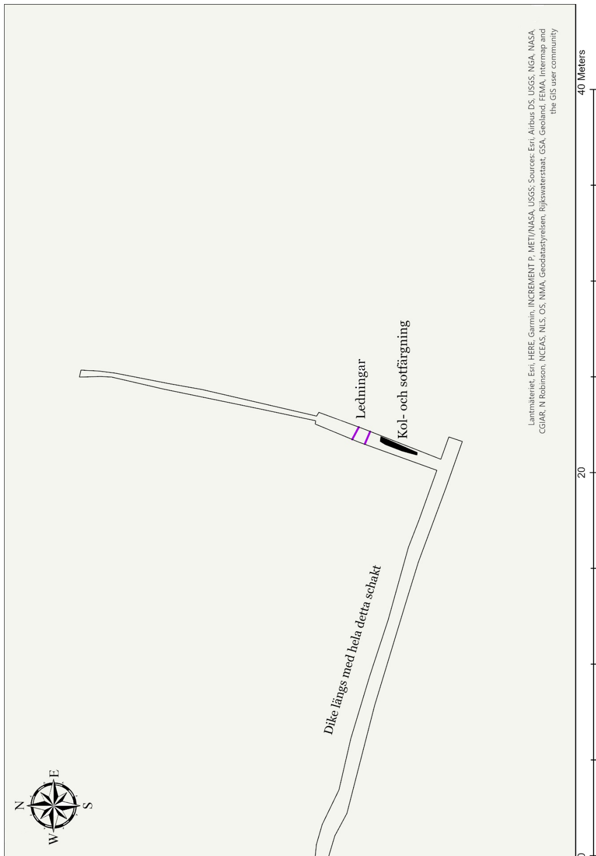
Figur 23. Den östra delen av det lilla schaktet. I det öst-västra schaktet fanns ett igenfyllt dike. Under vägen framkom en äldre markyta samt ledningar. © Esri
