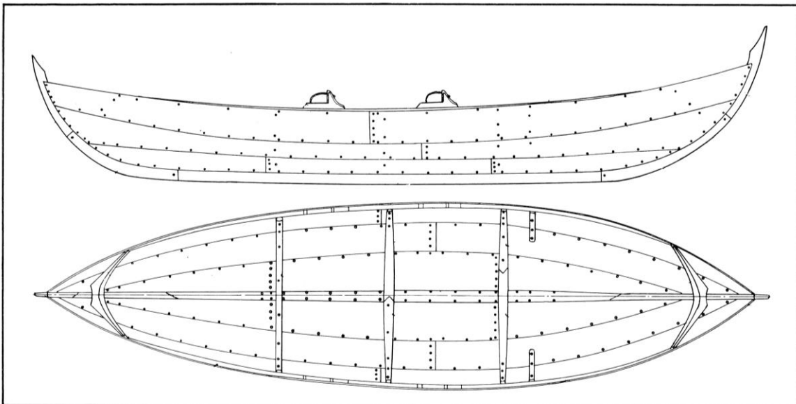
Hardangerbåt, oppmålingsteikning av Bernhard Færøyvik, henta frå «Vestlandsbåtar».
